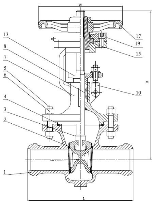
EN 12627 Fig1 tn≤4mm DN50 - DN80
