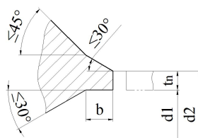
EN 12627 Fig1 tn≤4mm DN50 - DN80
